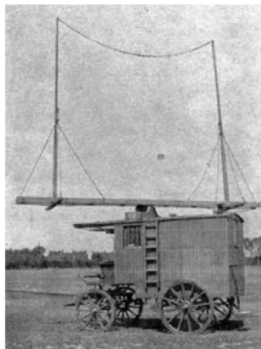
方探システム(1920年頃)とモービル(?)方探アンテナ(1918年頃)
