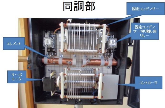
JF1VNR 7~21MHz 大口径MLAの試作品：下部のコントロール・ボックス内部
