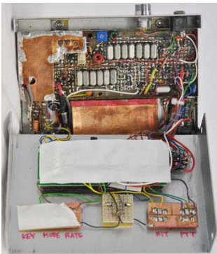
JAIUHIJの6mSSB/CWトランシーバ
