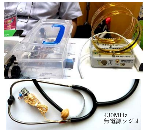
J1IHZ 片倉さんのエアバンド無電源ラジオ(左上)
